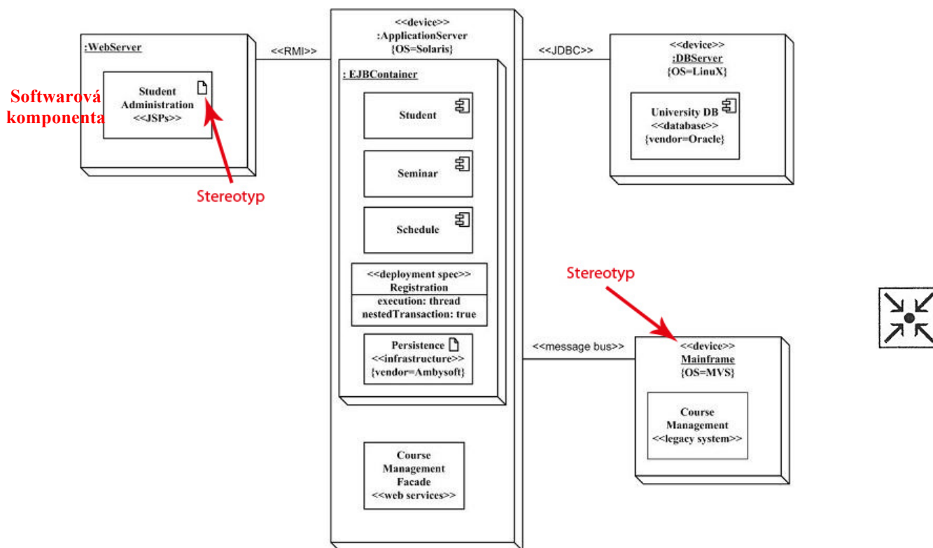
Obr. 7-5: Diagram nasazení univerzitního informačního systému [Am02].
