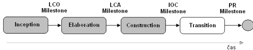
Obr. 5-10: Fáze Transition
