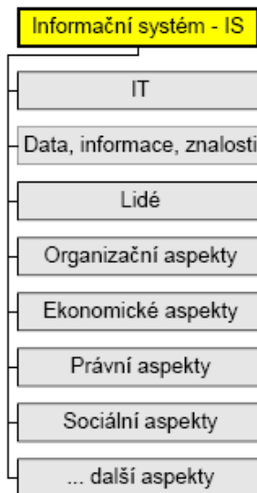
Obr. 2-2: Aspekty IS
