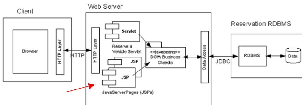
Obr. 7-6: Diagram komponent
