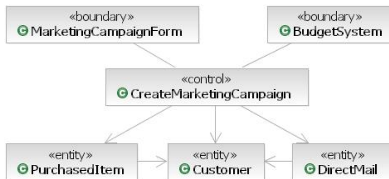
Obr. 6-14: Entity-Control-Boundary model (zdroj [OpenUP]).
