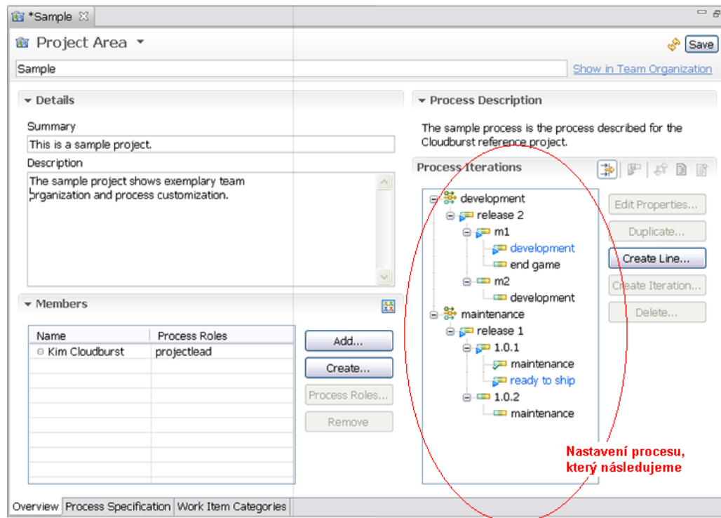
Obr. 6-36: Process View - definice procesu, který tým následuje, zdroj [Jazz].
