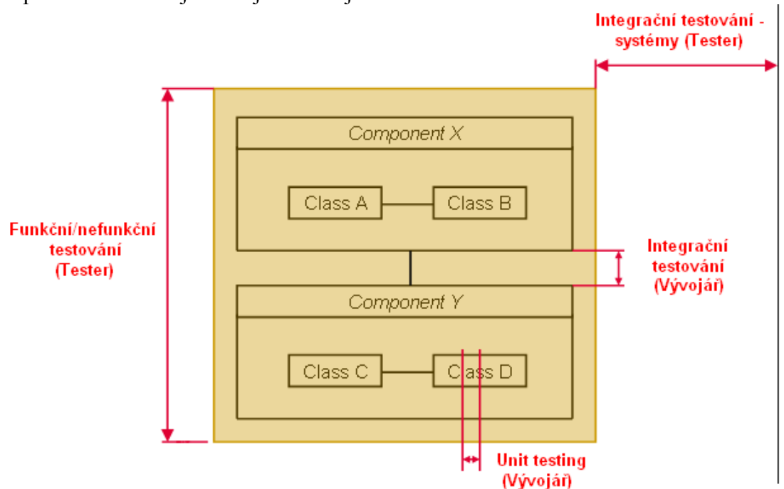
Obr. 6-21: Předmět testování
