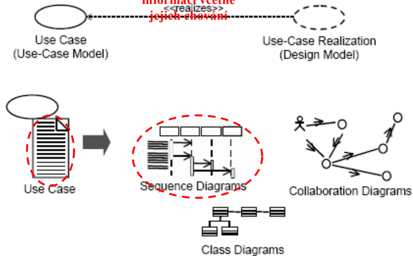
Obr. 6-13: UC realizace
