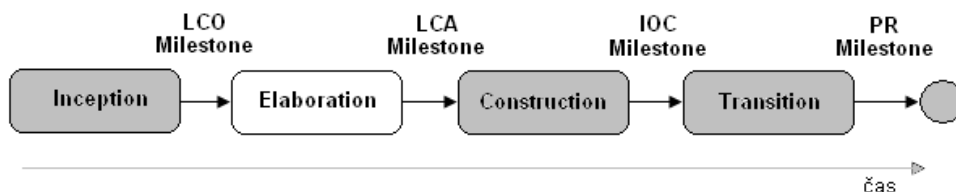
Obr. 5-5: Fáze Elaboration
