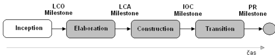
Obr. 5-4: Fáze Inception
