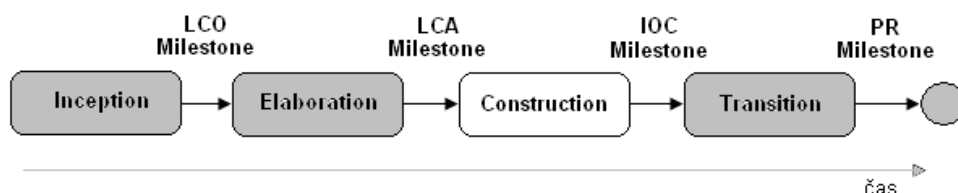
Obr. 5-8: Fáze Construction
