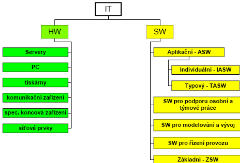
Obr. 2-1: Rozdělení IT
