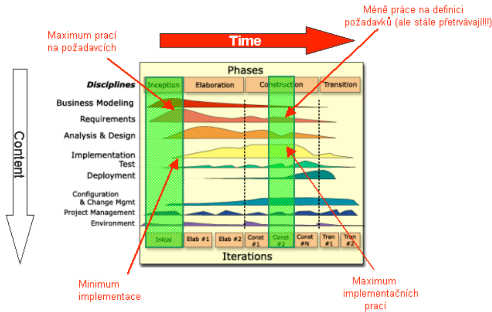
Obr. 5-2: Dvojměrný model RUP - fáze a disciplíny
