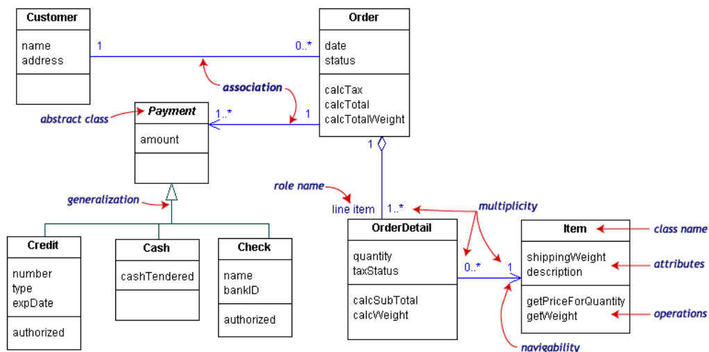
Obr. 7-8: Ukázka použití diagramu tříd (Zdroj: [Mi09])
