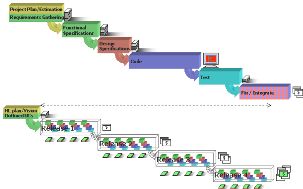
Obr. 5-1: Tradiční vs. iterativní model vývoje
