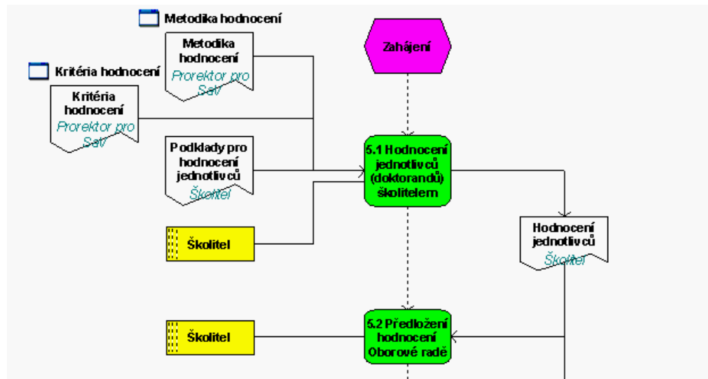
Obr. 6-2: Příklad notace procesu pomocí ECP
