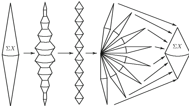
Fig. 124 A p^k -fold map \Sigma X \rightarrow \Sigma X
