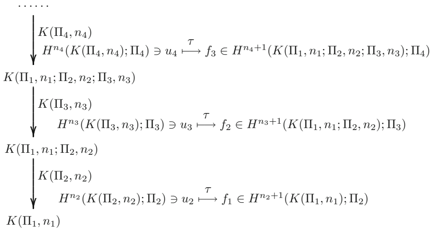
Fig. 133 The Postnikov tower
